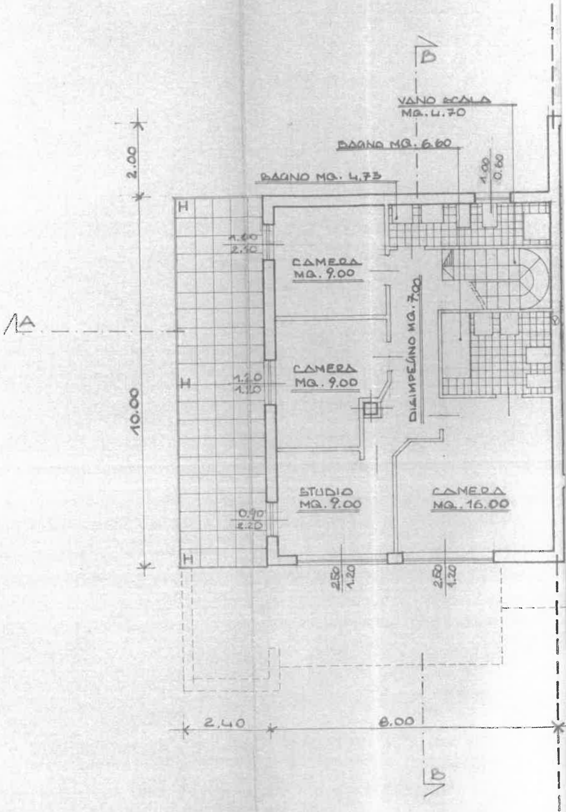
PIANTA ZONA NOTTE APPARTAM. A1
