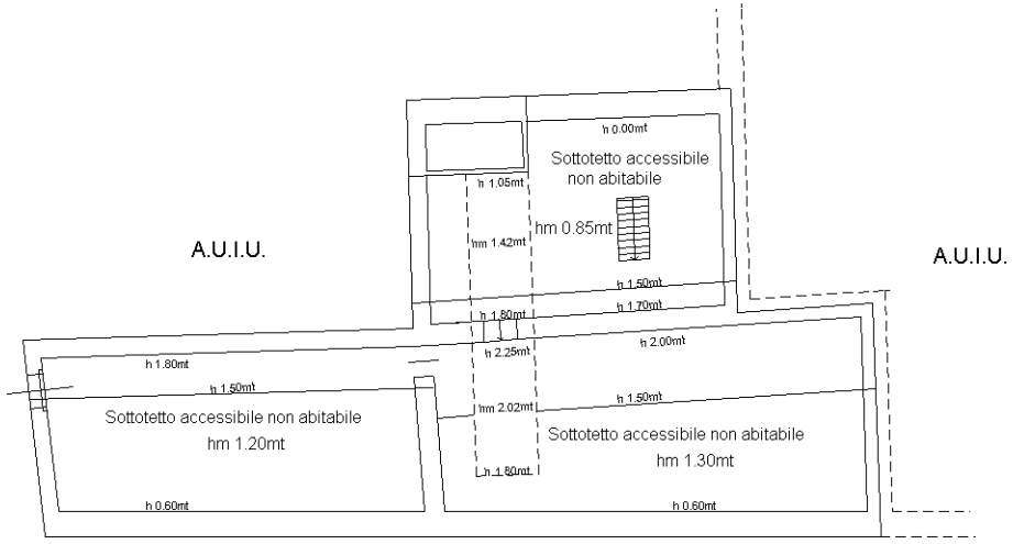
PIANO TERZO (SOTTOTETTO)
